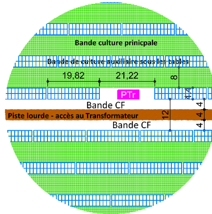
Détail - 1/1000
