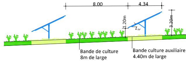
Détail table - 1/200
